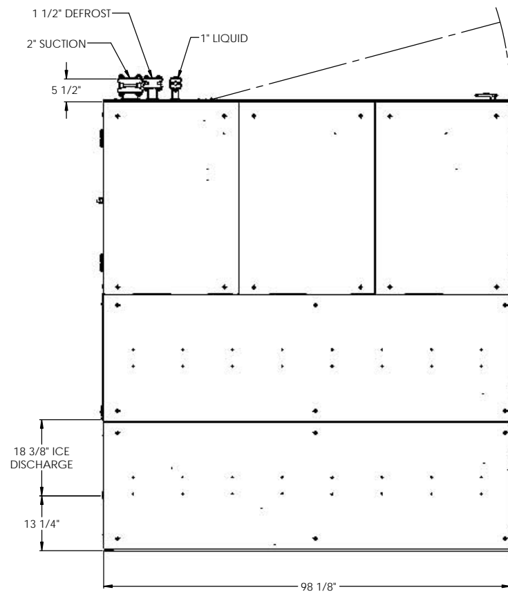
END ELEVATION
